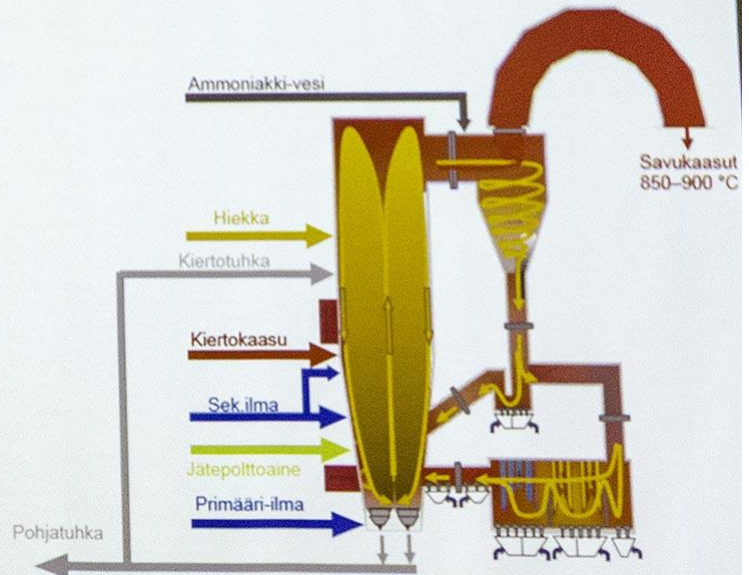
Kuva 4. Leijukattila.
